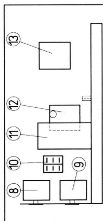
Schaltkastenkonsole
